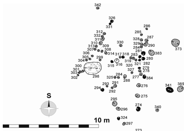
Obr. 136 Turnov-Maškovy zahrady, plocha C: půdorys CB3. Černě vyznačeny objekty s keramikou lužické kultury. Podklad MČR Turnov. – Abb. 136 Turnov-Maškovy zahrady, Fläche C: Grundriß CB3. Schwarz sind die Objekte mit Keramik der Lausitzer Kultur markiert. Unterlage Museum des Böhmisches Paradieses Turnov.
