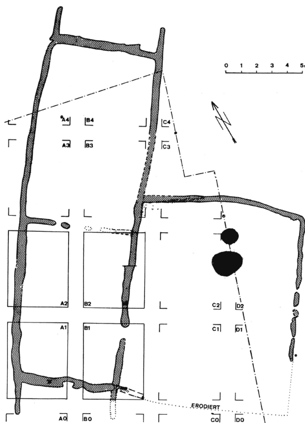
Obr. 89 Wetzleinsdorf, Rakousko: půdorys domu lengyelské kultury, zúžení žlabu snad indikuje vchod. Podle O. Urbana (1980, Taf. 3:1). – Abb. 89 Wetzleinsdorf, Österreich: Hausgrundriß der Lengyel-Kultur, die Verengung des Wandgräbchens bedeutet wohl die Stelle des ehemaligen Eingangs. Nach Urban 1980, Taf. 3:1.
